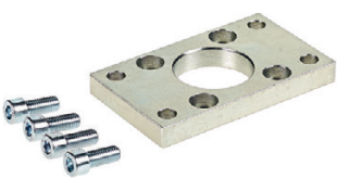
Flange ISO
